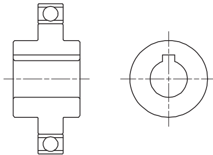
Starre Ausführung Rigid type
