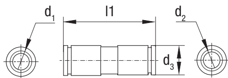
Typ A (gerade Ausführung)
