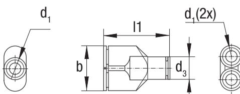
Typ D (Y-Ausführung)
