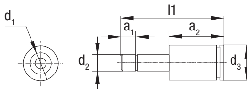
Typ B (reduzierte Ausführung)
